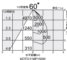
照明率表 P.945-B-
