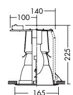
150 埋込穴
