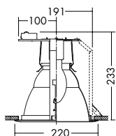
200 埋込穴
