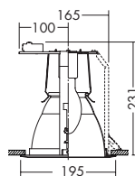
175 埋込穴
