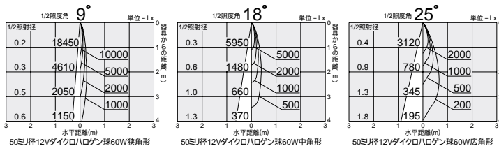
照明率表 P.942-F-1 照明率表 P.942-F-2 照明率表 P.942-F-3
