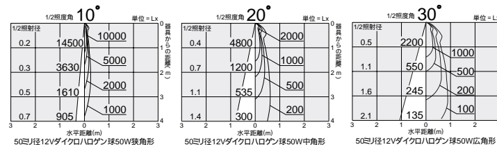
照明率表 P.942-F-4 照明率表 P.942-F-5 照明率表 P.942-F-6
