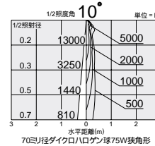
照明率表 P.949-A-
