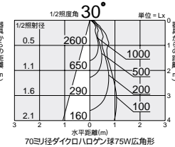
照明率表 P.949-A-
