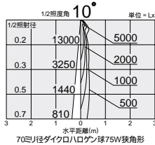
照明率表 P.949-A-
