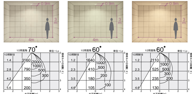
照明率表 P.945-D-2
