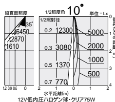
12V低内圧ハロゲン球・クリア75W
