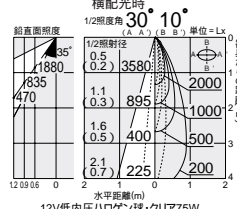
12V低内圧ハロゲン球・クリア75W
