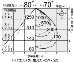
照明率表 P.945-F-
